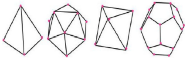
Figura 4.2: Sólidos platónicos
